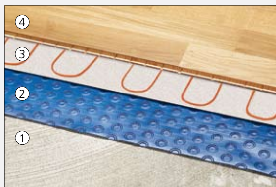
1. Beton 2. Platon Stop Original 3. Varmefolie med udligningsunderlag 4. Overgulv
